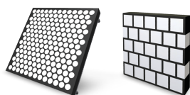
Revestimientos cerámicos antidesgaste para transportadores de minería X-Wear
